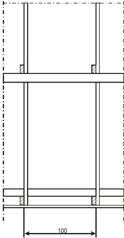
Detaliu A-A
